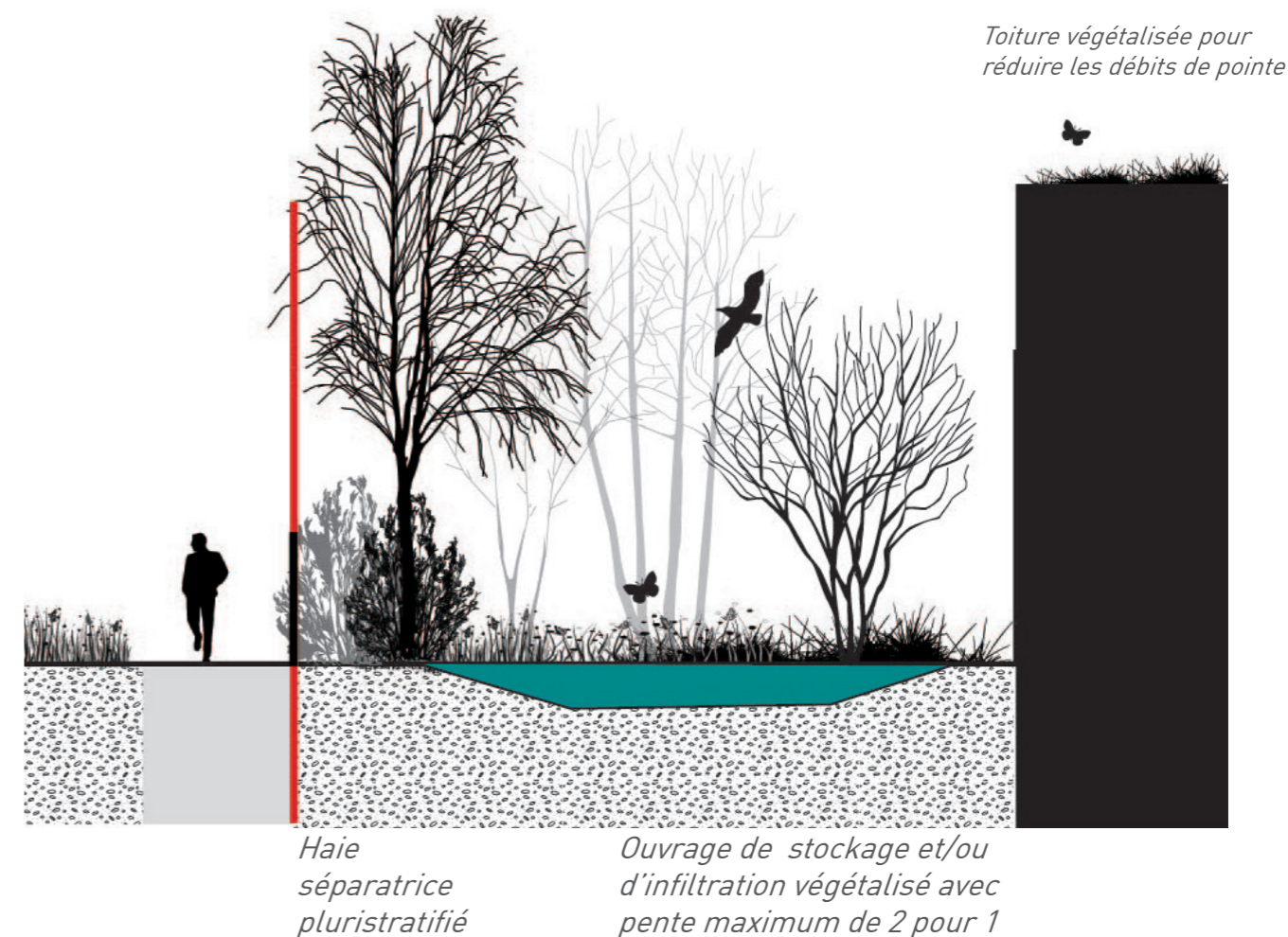
Principes d'intégration d'un bassin et de végétalisation
