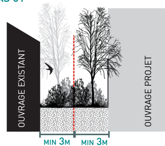
> Cas d'un projet de surface d'exploitation en limite
