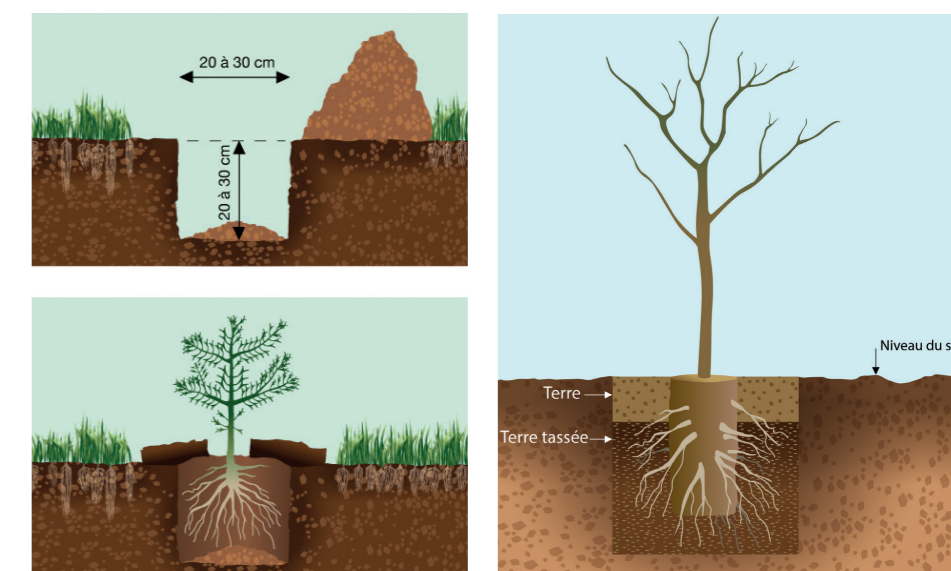
Plantations des haies : cas d'une plantation en godet dans un sol déjà constitué
