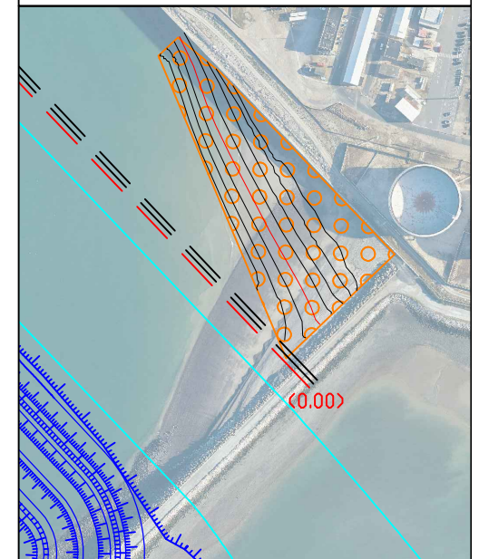
Déplacement des galets Schéma de principe
